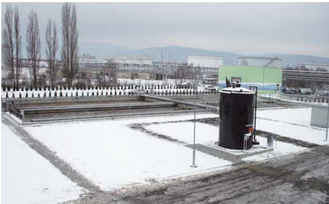
Nová ČOV Litvínov s kapacitou 36 000 ekvivalentních obyvatel je v ročním zkušebním provozu.
