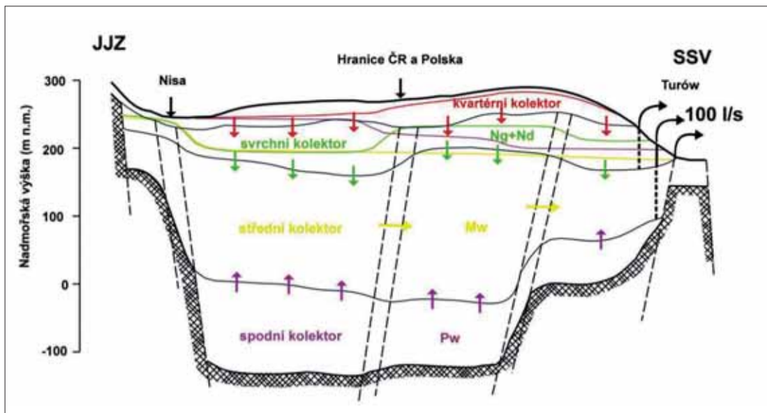
Schématický hydrogeologický profil centrální strukturou hradecké pánve - barevnými šipkami je naznačen směr přetékání.
